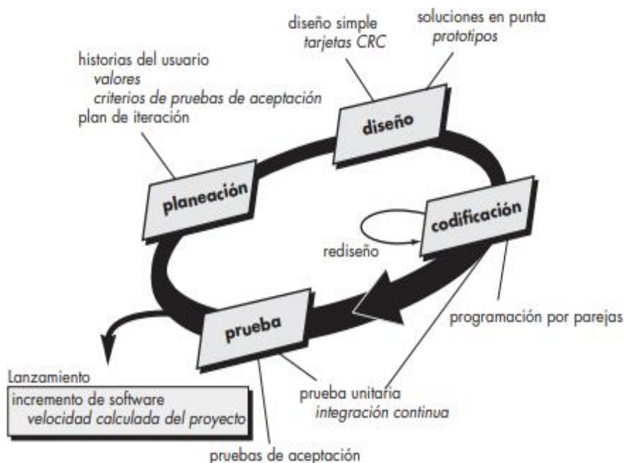
Figura 4.1. Esquema del Proceso XP
